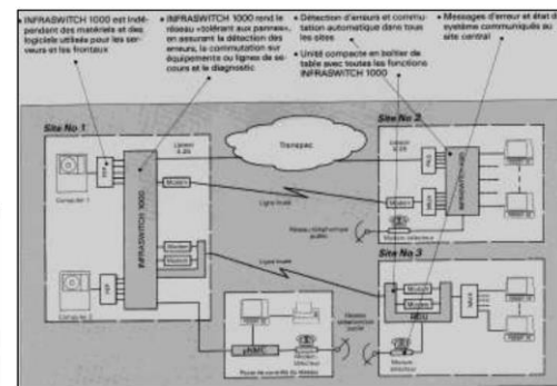
Sécurisation des réseaux/Infraswitch
