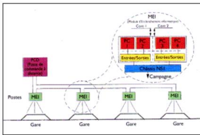
Architecture du PIPC
